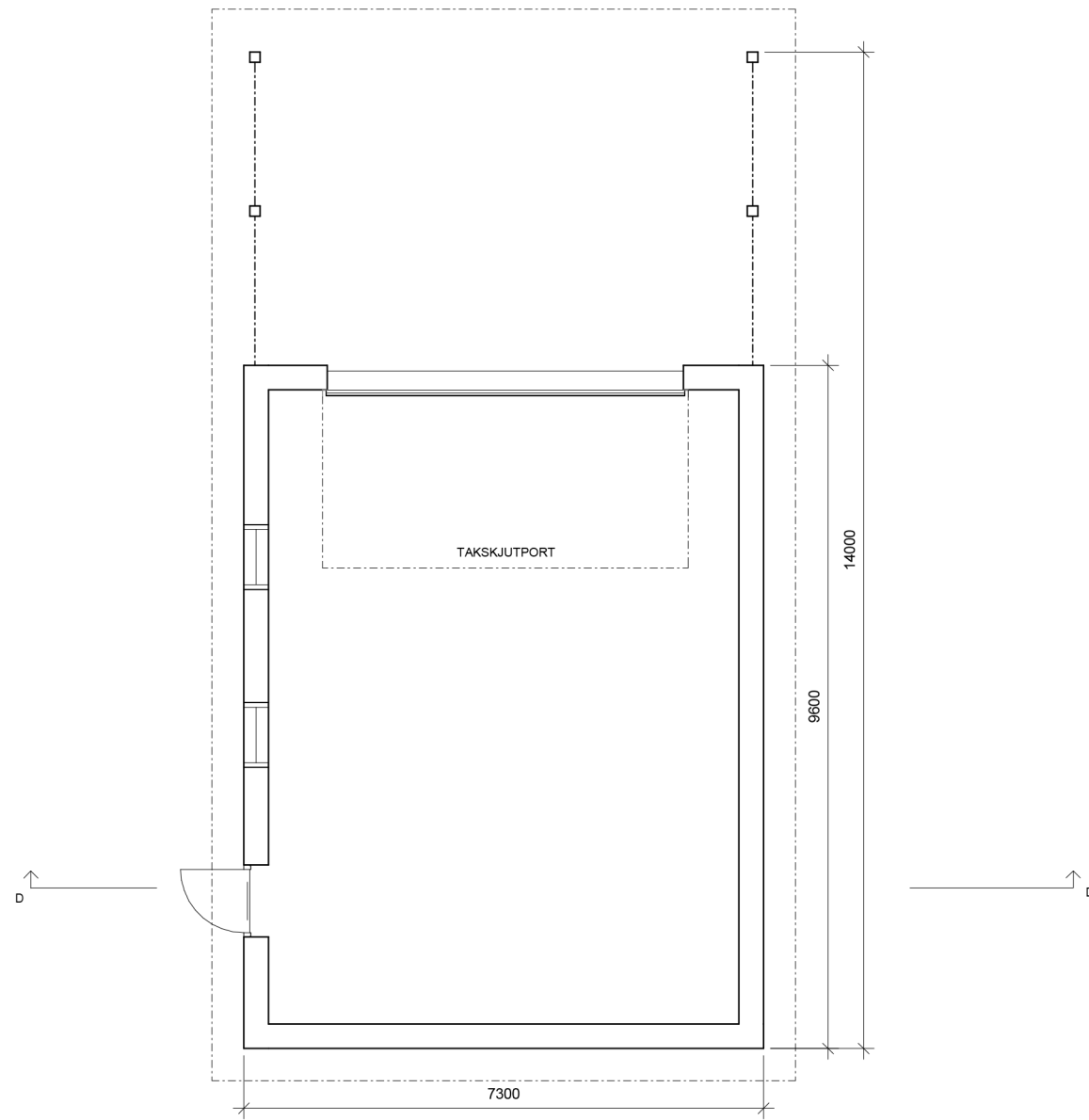
PLAN 1:100
