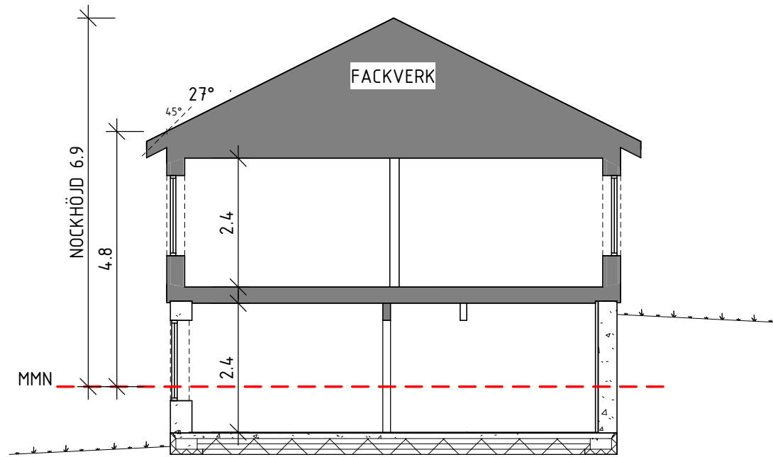
SEKTION A-A
