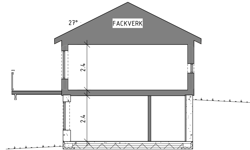
SEKTION B-B
