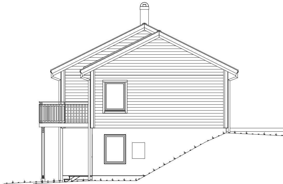
FASAD MOT HÖGER
