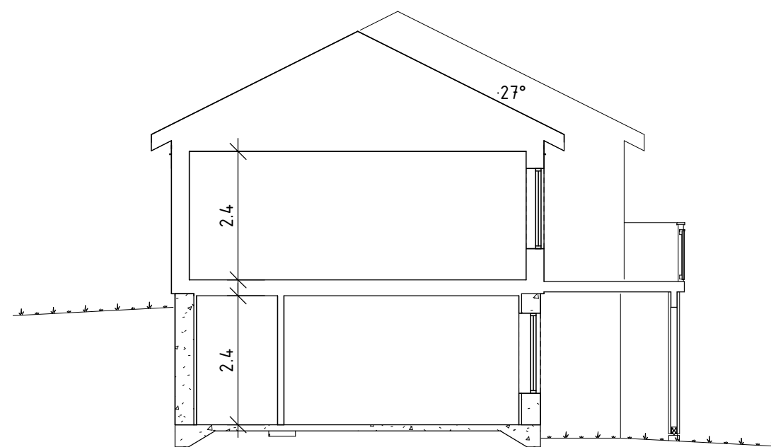
SEKTION B-B
