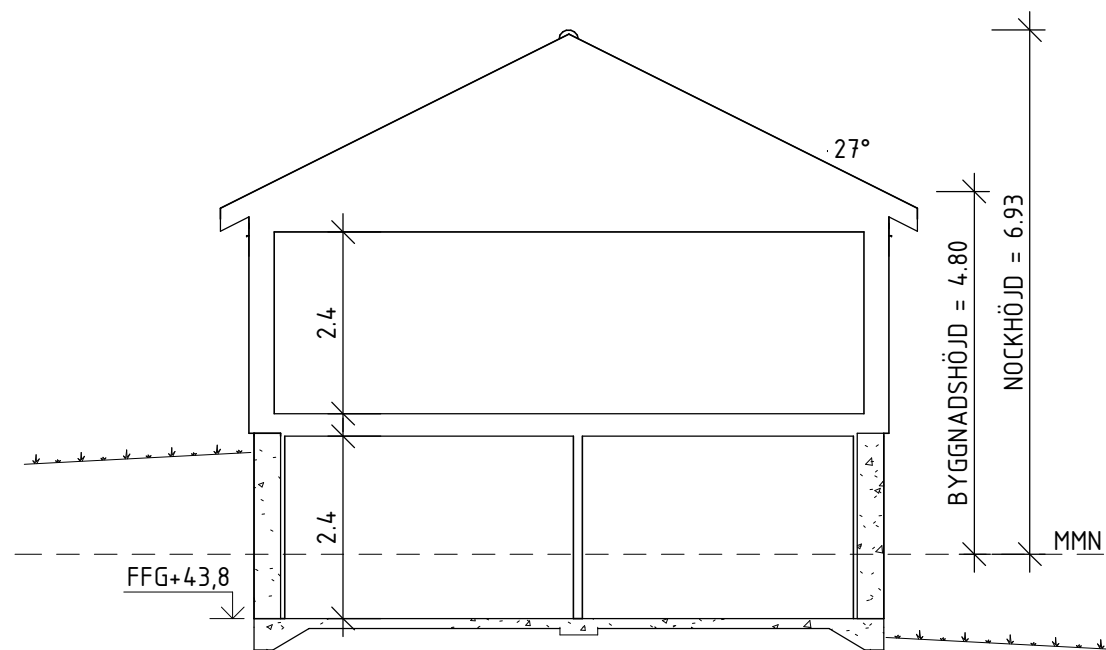
SEKTION A-A
